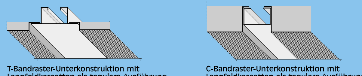
T-Bandraster-Unterkonstruktion mit Auflagekassetten als Langfeldkassetten
